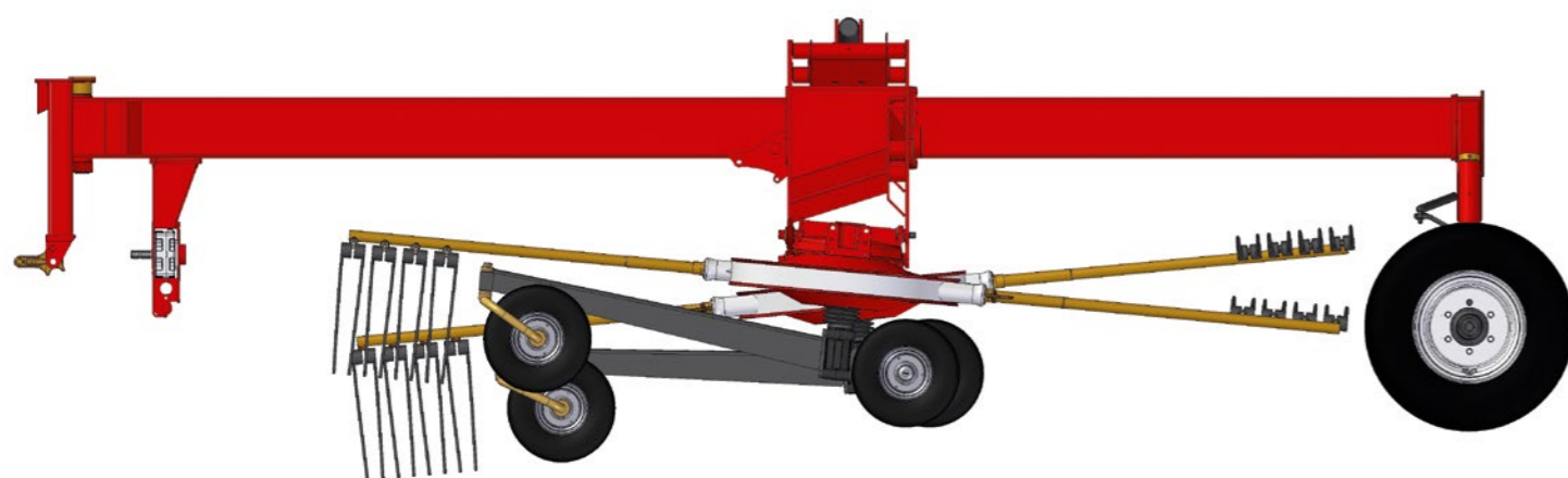
Opatentowane zawieszenie wirników z pełnym zastosowaniem przegubów Kardana
